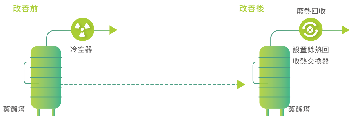
蒸餾塔塔頂餘熱回收
