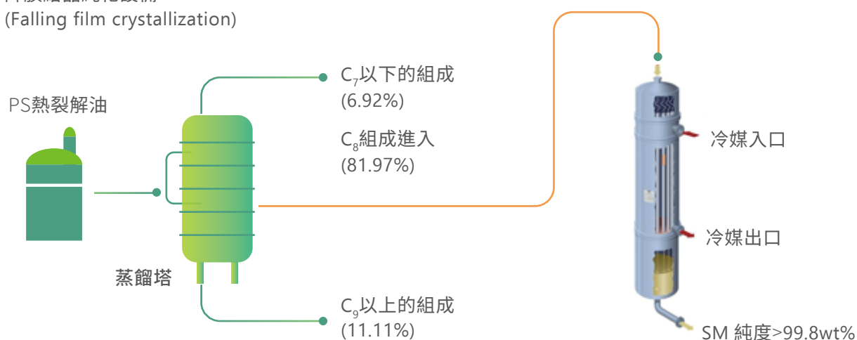
降膜結晶純化設備
